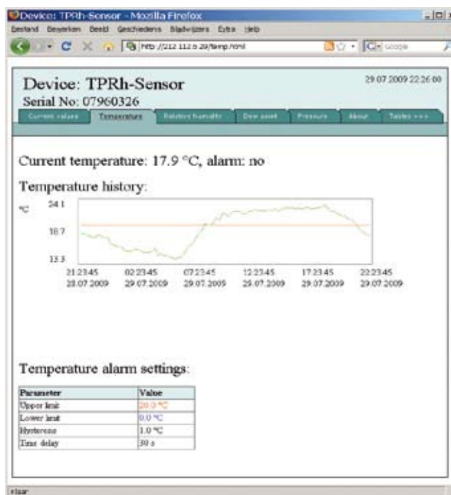
Voorbeeld van een webpagina die een trend van de laatste 300 temperatuur meetwaarden weergeeft.
